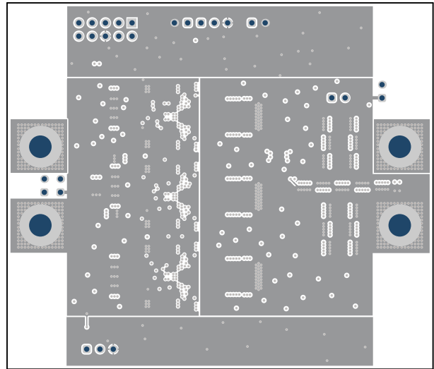
Figure 5-4. Layer 3
