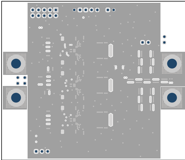
Figure 5-9. Layer 8
