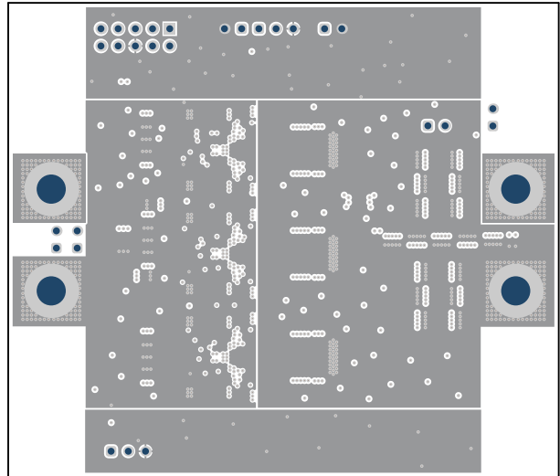
Figure 5-8. Layer 7
