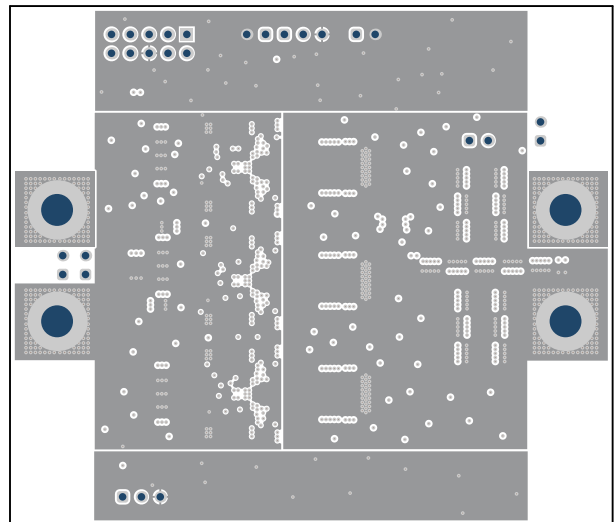
Figure 5-6. Layer 5
