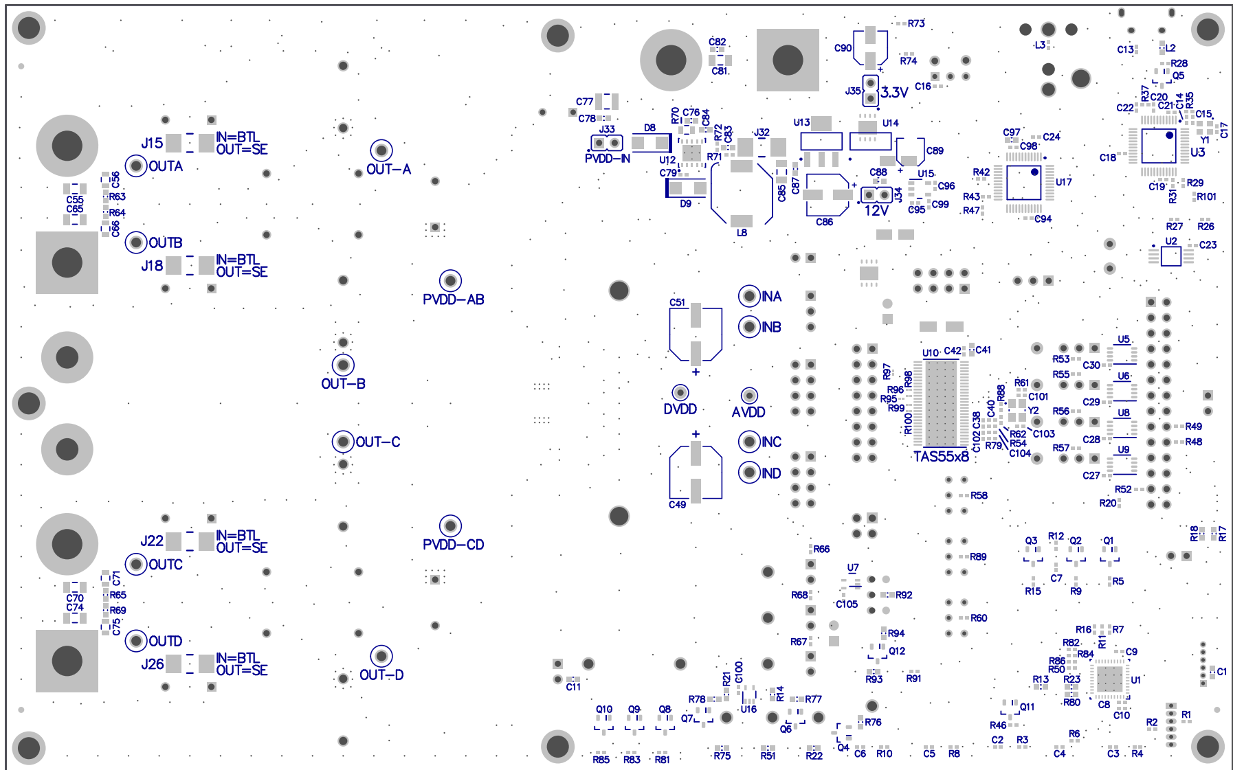
Bottom Overlay
