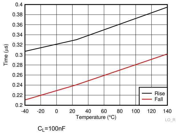
Figure 6-26. LO Rise & Fall Time
