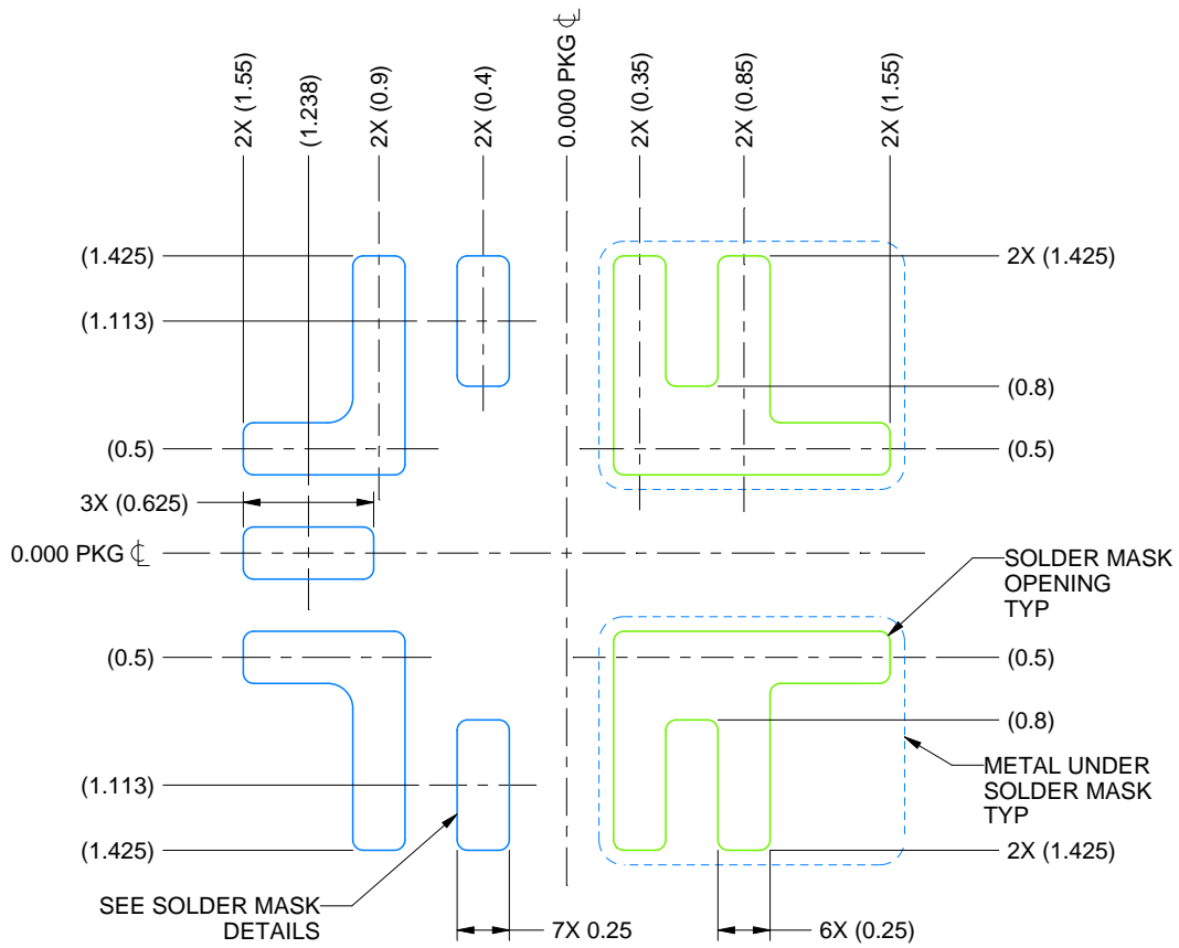
LAND PATTERN EXAMPLE SCALE: 25X
