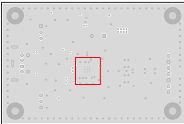
Figure 21. Bottom Layer
