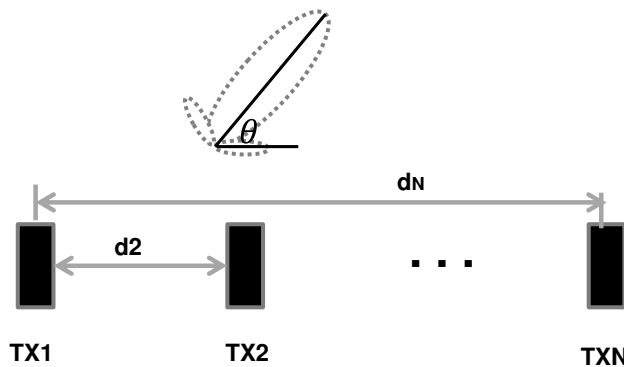
図 9. TX Array for Beamforming
