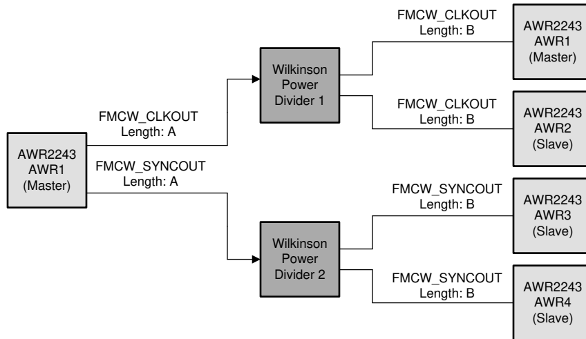
図 3. 20 GHz LO Distribution Block Diagram
