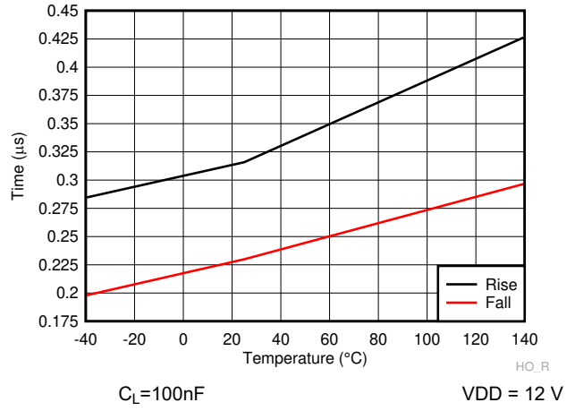
6-21. HO Rise & Fall Time
