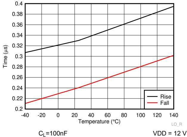
6-20. LO Rise & Fall Time
