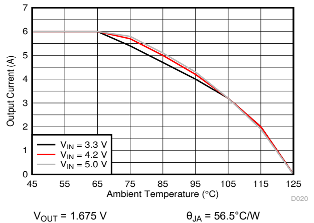
9-11. Thermal Derating
