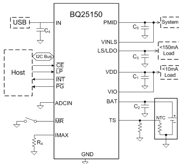
簡略回路図
