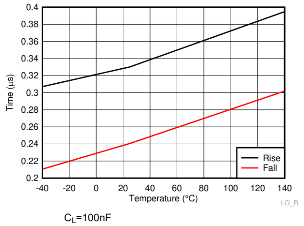
6-26. LO Rise andamp; Fall Time
