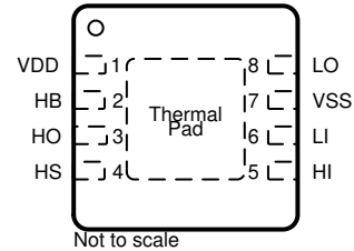
图 5-2. DRM Package 8-Pin SON Top View
