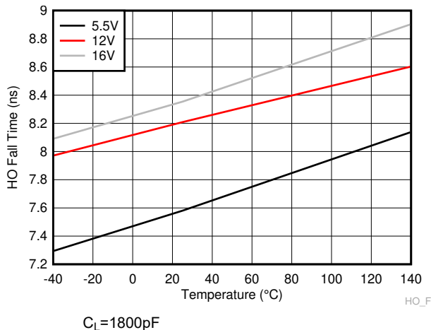
6-25. HO Fall Time
