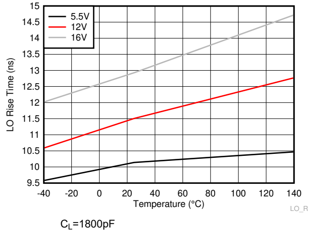
6-22. LO Rise Time
