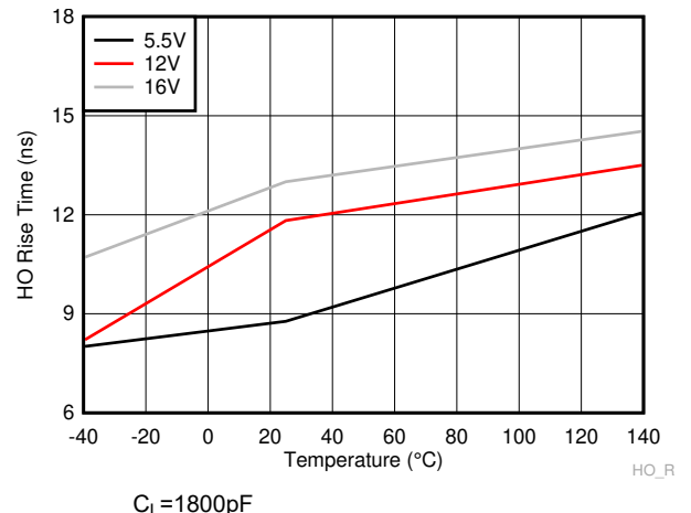
6-24. HO Rise Time
