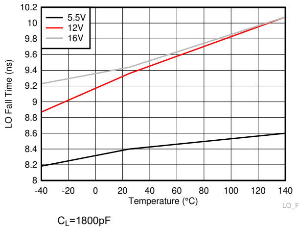
6-23. LO Fall Time
