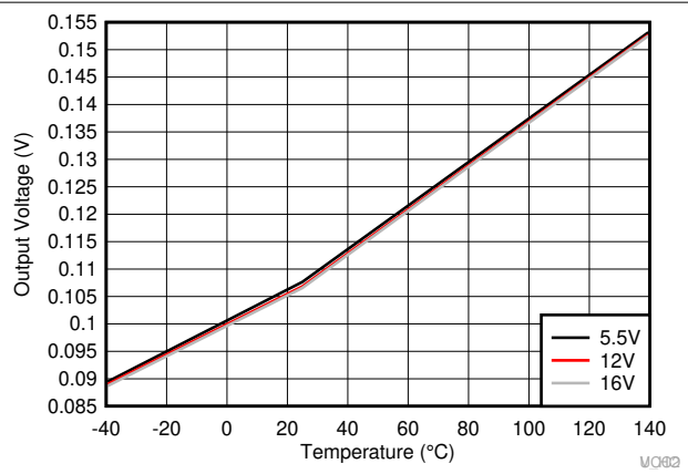
6-18. LO Low Output Voltage ( V_{LOL} )
