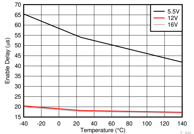
6-12. Enable Delay
