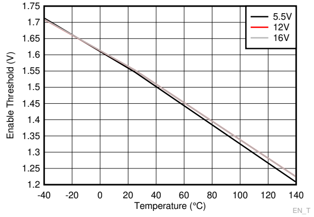
6-10. Enable Threshold
