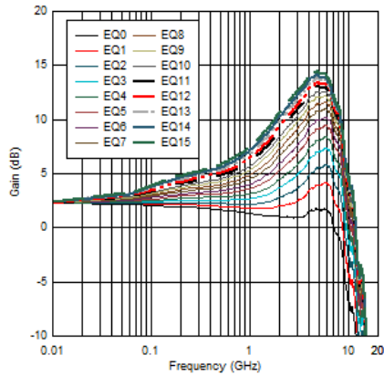
图 5-3. USB RX1 EQ Settings Curves
