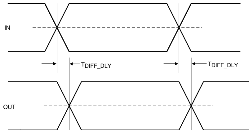
图 6-3. Propagation Delay
