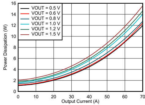
图 5-7. TPSM8D6C24 Power Dissipation vs Output Current
