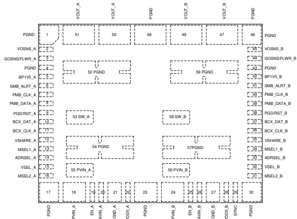
図 4-1. 59-Pin QFM-MOW Package (Top View)
