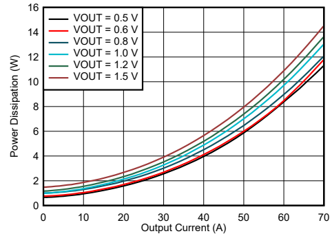
图 5-8. TPSM8D6C24 Power Dissipation vs Output Current
