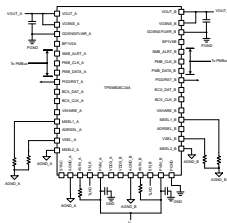
アプリケーション概略図
