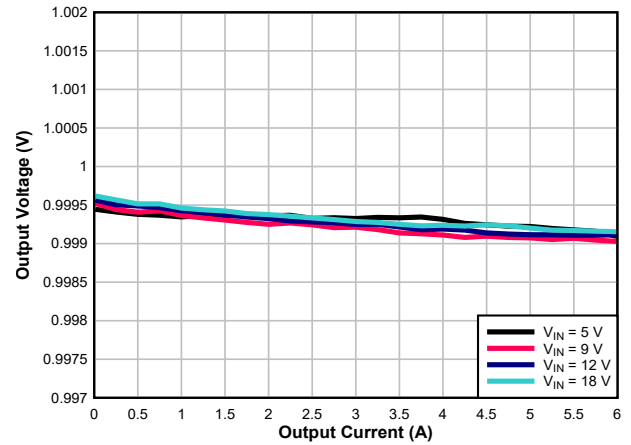
図 7-5. Load Regulation
