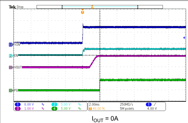
図 7-13. VIN Start-Up
