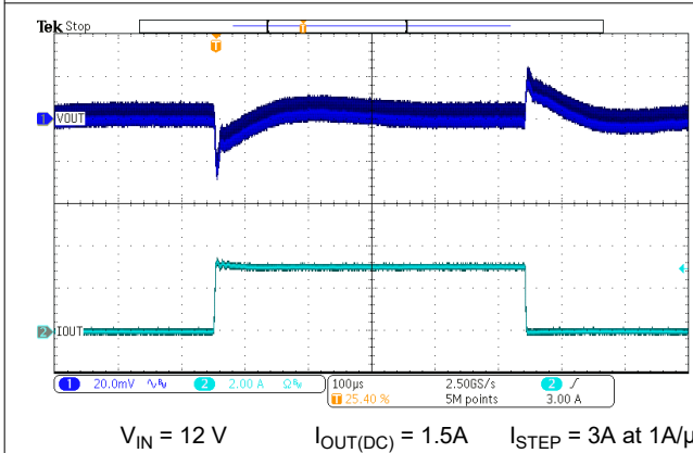
図 7-8. Load Transient
