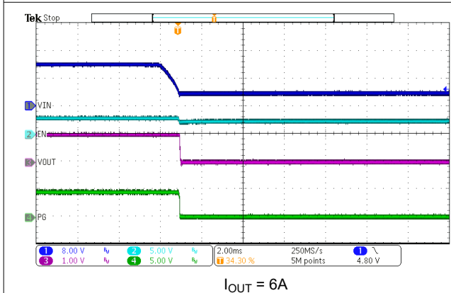
図 7-14. VIN Shutdown
