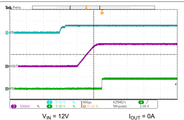
7-9. EN Start-Up – No Load
