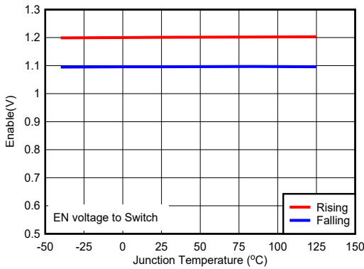
图 5-5. Enable Voltage
