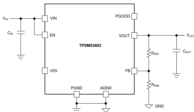
概略回路図
