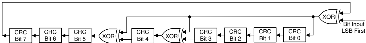
図 6-9. CRC Algorithm Diagram
