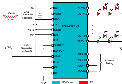
代表的なアプリケーションの図
