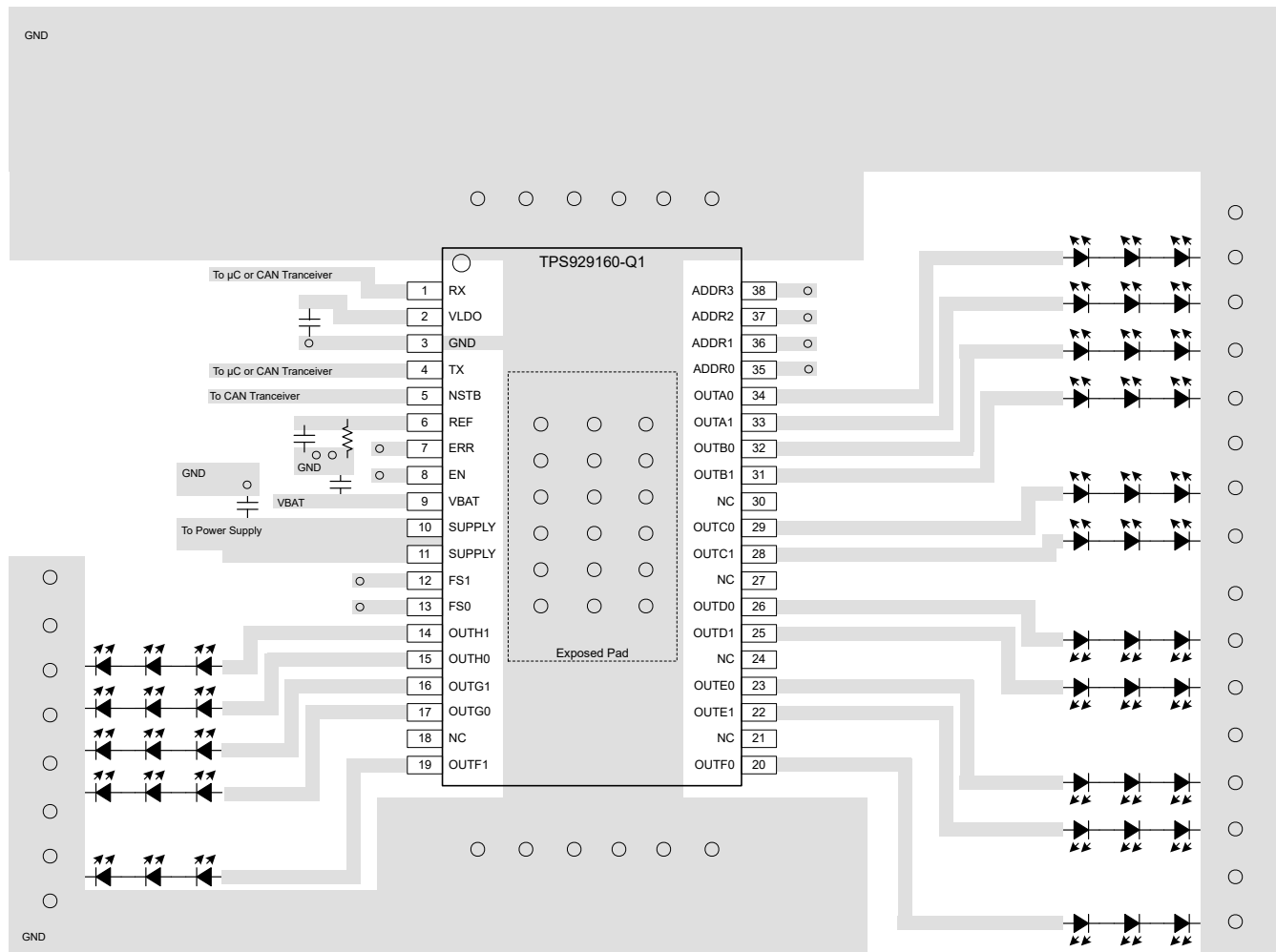
☒ 7-5. TPS929160-Q1 Layout
