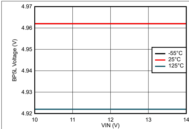
7-1. BP5L Output Voltage vs VIN Voltage
