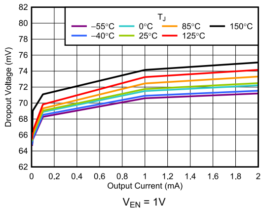
图 5-7. Dropout Voltage vs I_{OUT}
