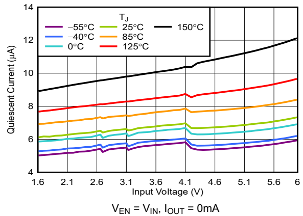
图 5-10. I_{GND} vs V_{IN}
