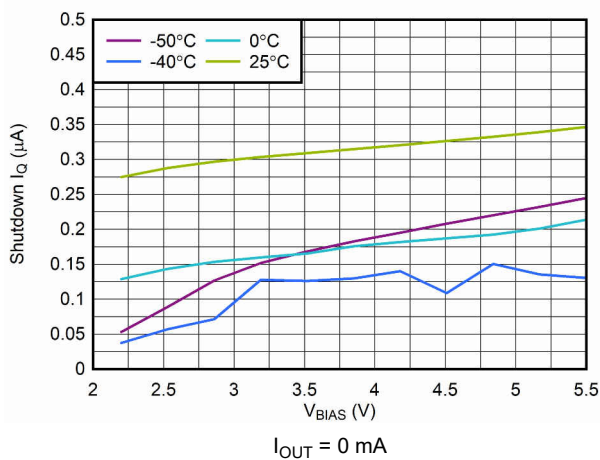
6-9. V_{\text{BIAS}} Shutdown I_Q vs V_{\text{BIAS}}
