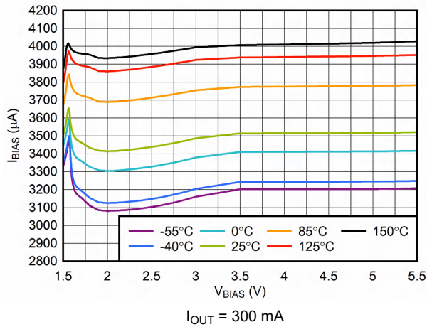
6-7. V_{\text{BIAS}} Input Current vs V_{\text{BIAS}}
