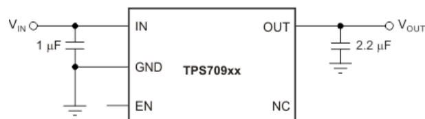
代表的なアプリケーション回路
