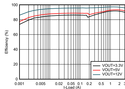
TPS62933 の効率 ( V_{IN} = 24V , f_{sw} = 500kHz )
