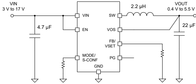
簡略回路図
