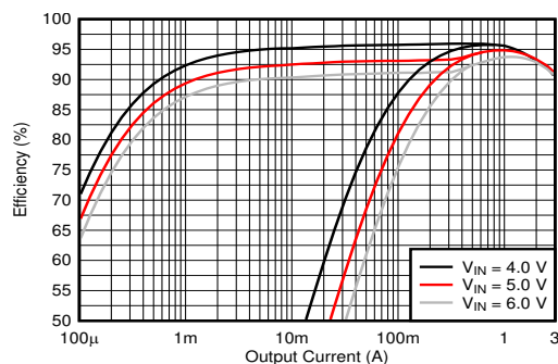
効率と I_{OUT} との関係、 V_{OUT} = 3.3\text{V}
