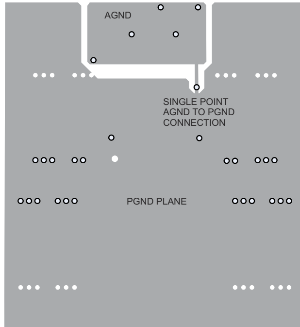
図 7-20. Mid Layer 1 Layout
