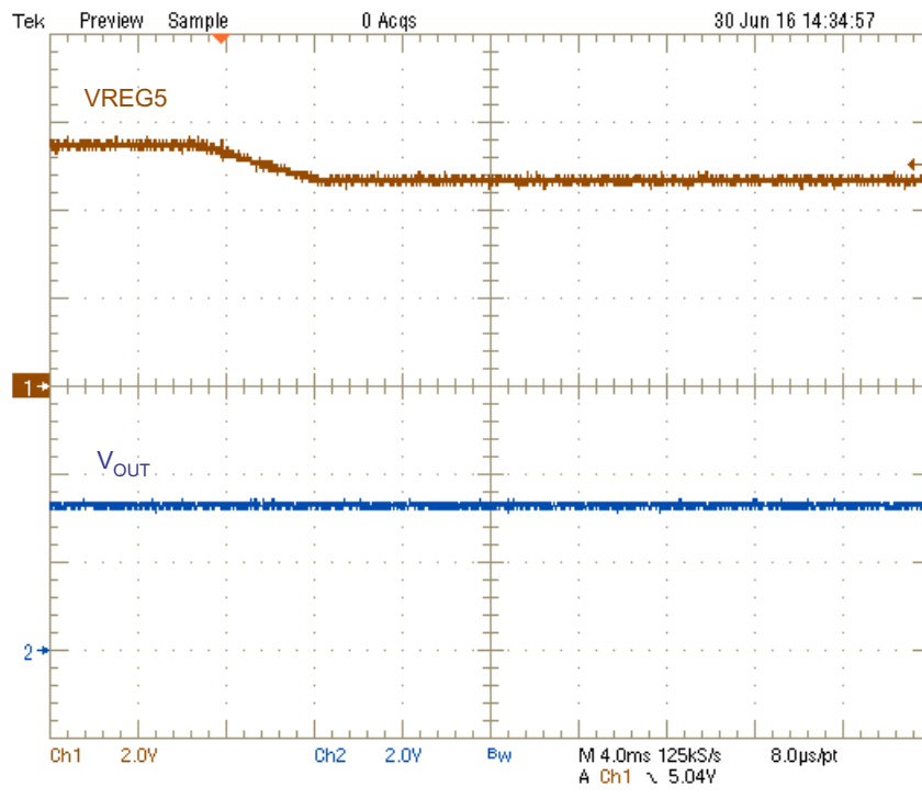
図 6-1. VREG5 Transition
