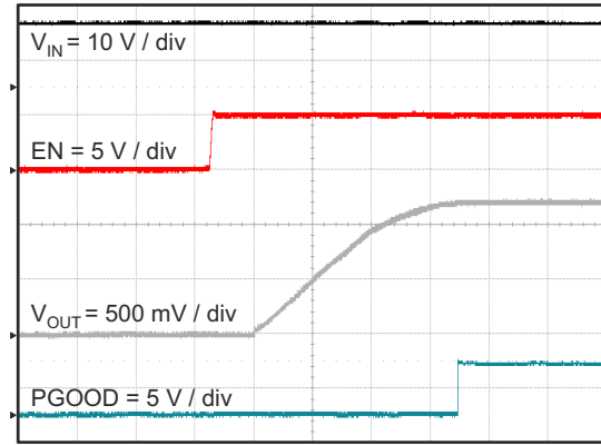
図 7-15. Start Up Relative to EN Rising
