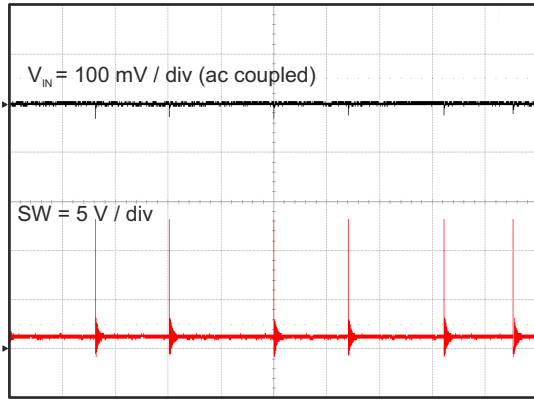
図 7-8. Input Voltage Ripple, I_{OUT} = 10 \text{ mA}
