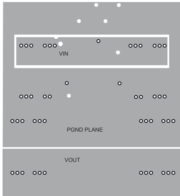
図 7-21. Mid Layer 2 Layout
