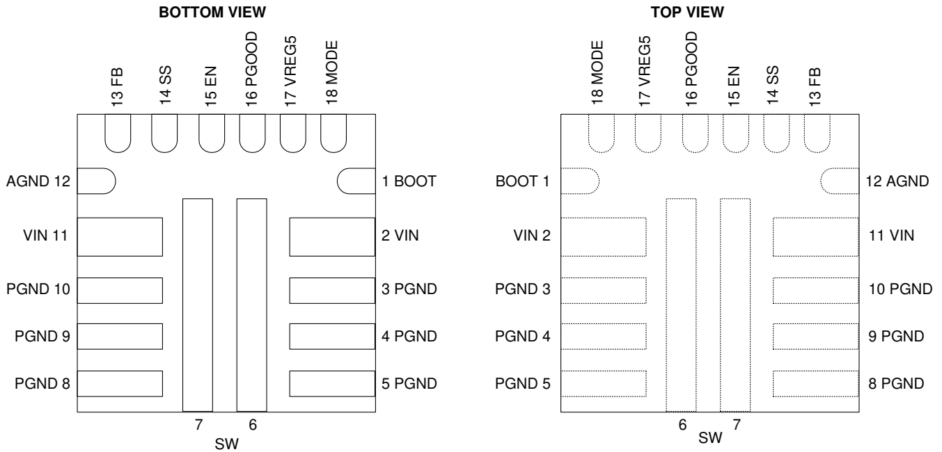
図 4-1. RNN Package, 18-Pin VQFN
