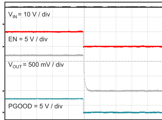
図 7-17. Shut Down Relative to EN Falling
