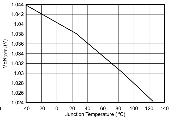
图 6-4. Enable Off Threshold Voltage
