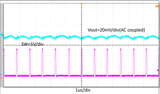
图 8-9. TPS564247 Output Voltage Ripple with 0.01-A Loading
