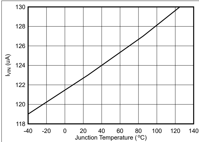
图 6-1. TPS564242 Quiescent Current
