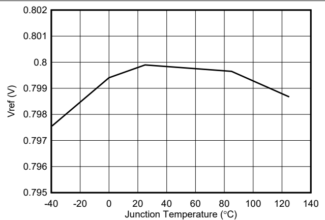
6-6. VREF Voltage
