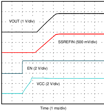
図 7-16. EN Start-Up
