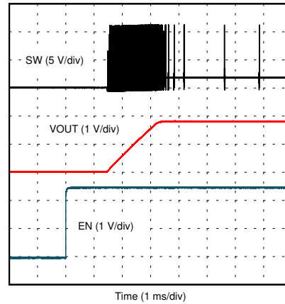
図 7-15. EN Start-Up
