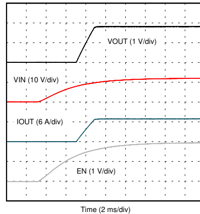
図 7-17. EN Start-Up – DCM
