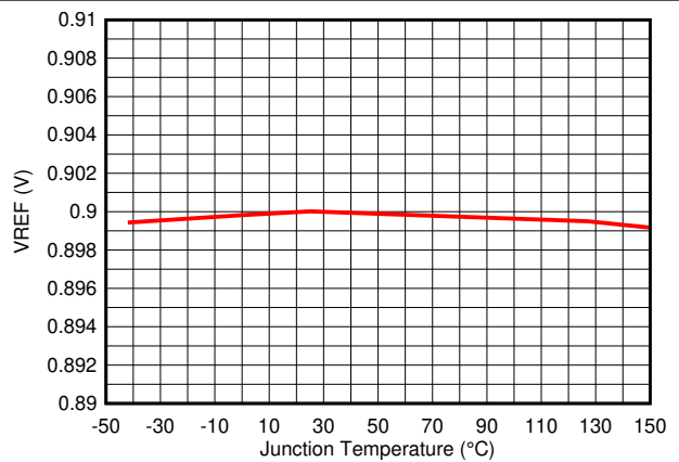
図 5-6. Vref
