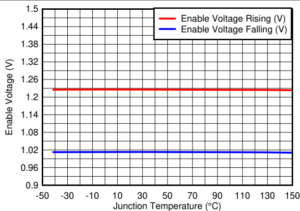
図 5-5. Enable Voltage
