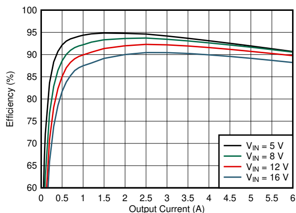
代表的な効率 ( V_{\text{OUT}} = 1.8\text{V} 、 f_{\text{sw}} = 600\text{kHz} )
