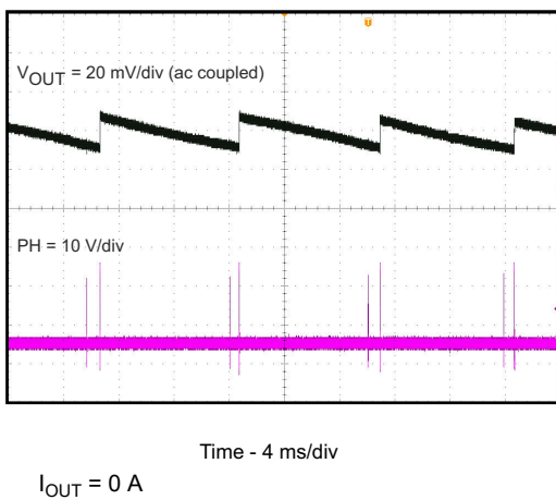
图 8-6. Output Voltage Ripple
