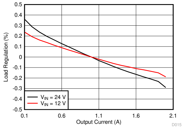
图 8-4. Load Regulation
