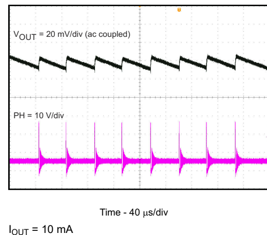
图 8-7. Output Voltage Ripple
