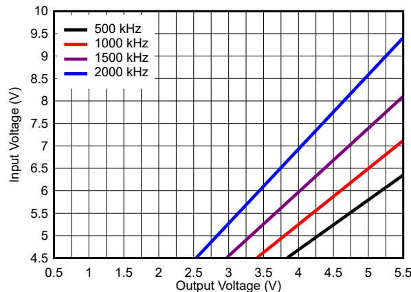
图 7-2. Minimum Input Voltage
