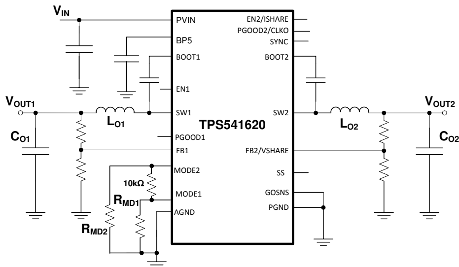
概略回路図 (デュアル出力)
