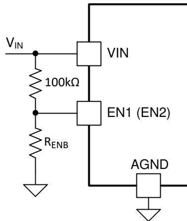
图 7-1. Enable ON/OFF Control
