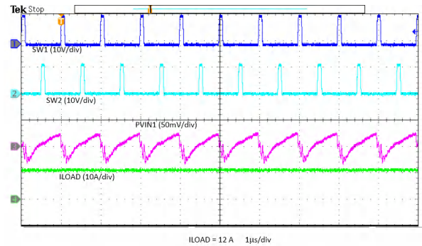
8-47. Input Ripple PVIN1 – 12-A Load
