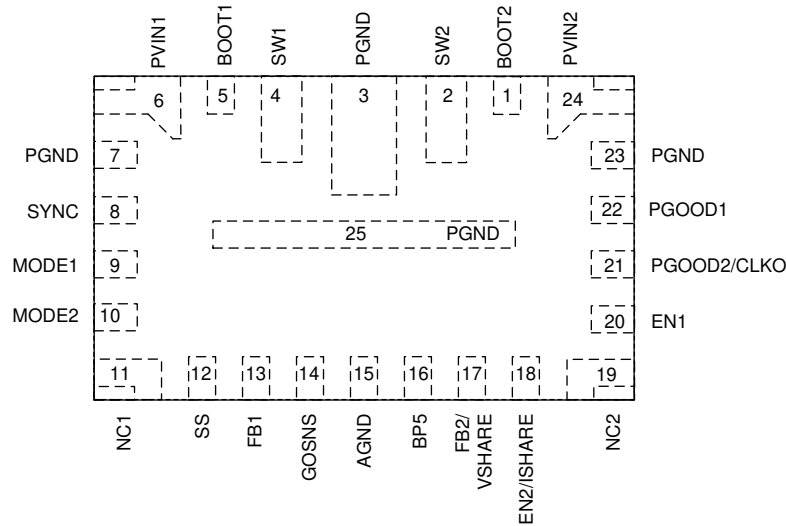
图 5-1. 25-Pin VQFN-HR RPB Package (Top View)
