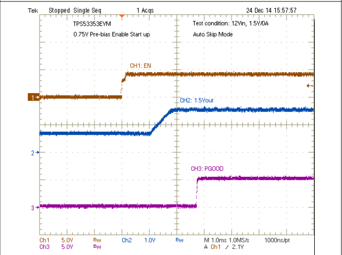
8-10. Output 0.75-V Prebias Turnon
