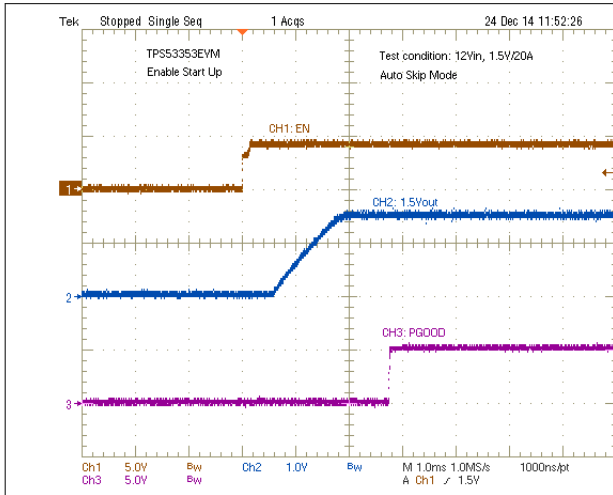
8-2. Enable Turnon
