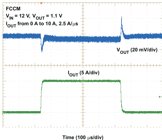
6-21. FCCM Load Transient
