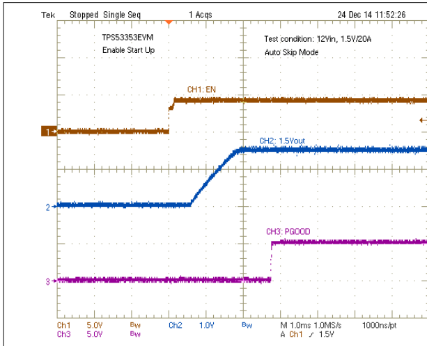
8-5. Enable Turnon
