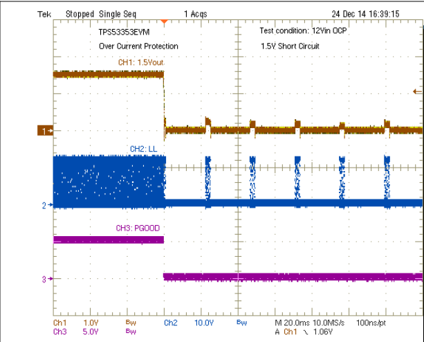
图 8-12. Output Short-Circuit Protection
