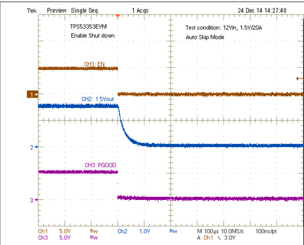
8-3. Enable Turnoff
