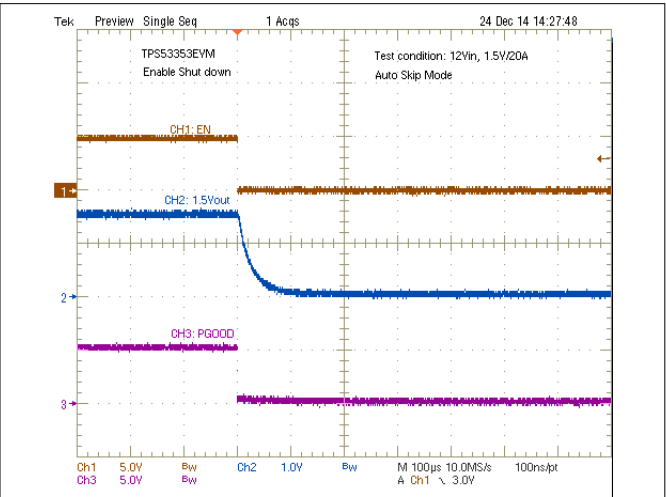
8-6. Enable Turnoff
