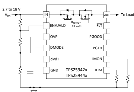
概略回路図
