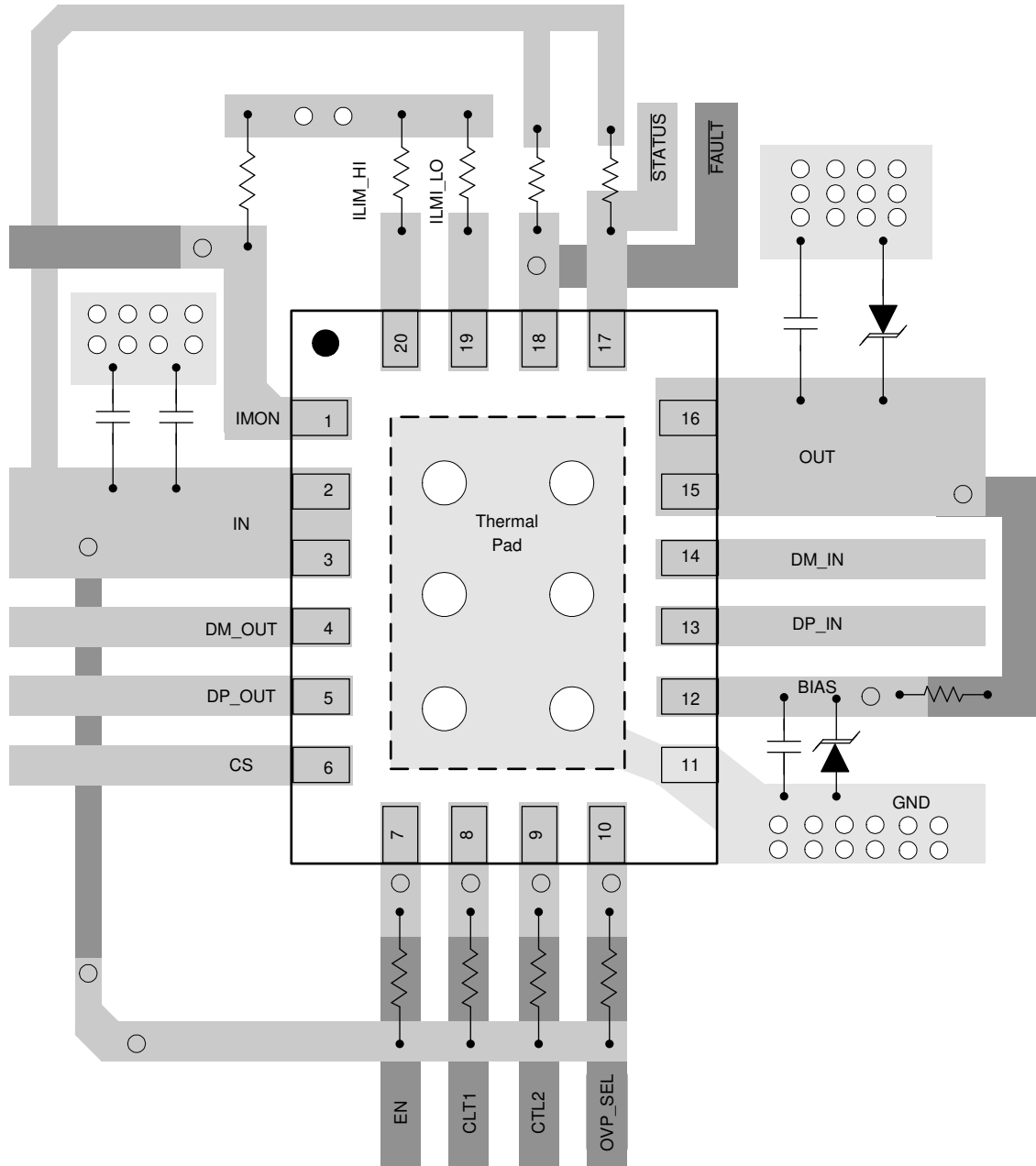
11-1. TPS254900A-Q1 Layout Diagram
