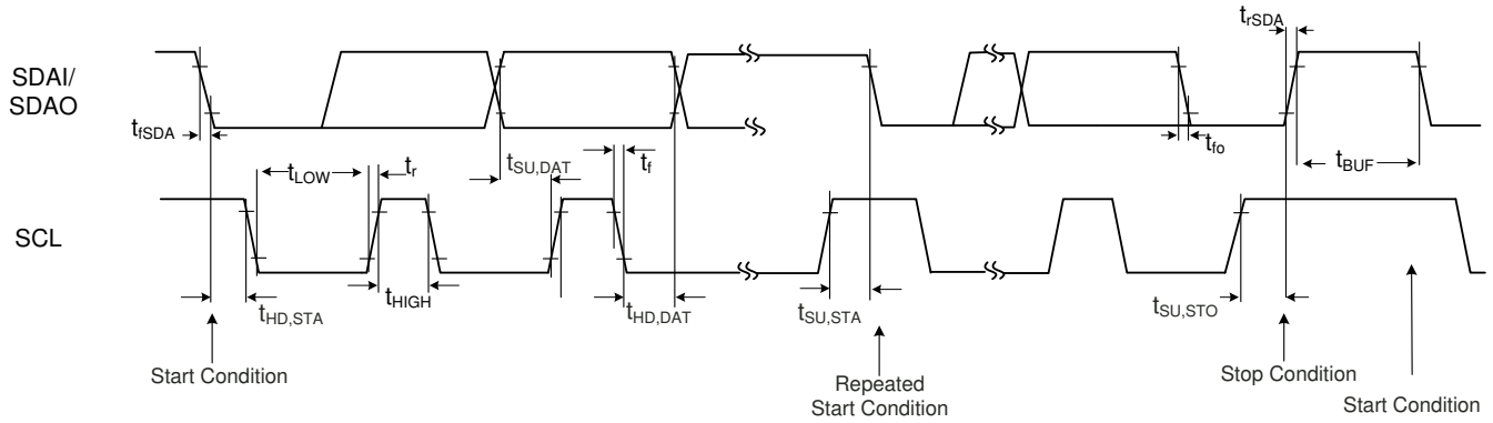
図 7-1. I 2 C Timings
