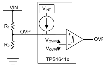
図 8-3. OVP Input in TPS1641x
