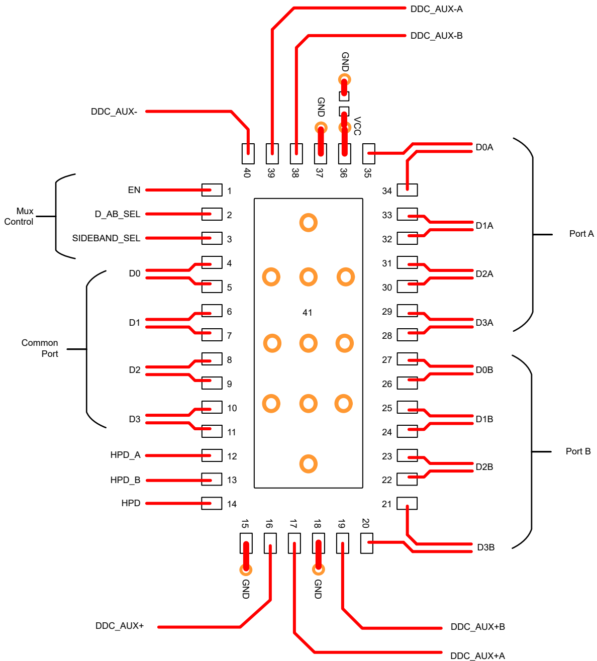
図 8-6. Layout Example
