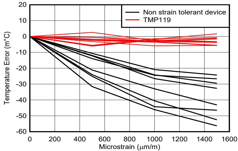
図 7-3. Strain Tolerance
