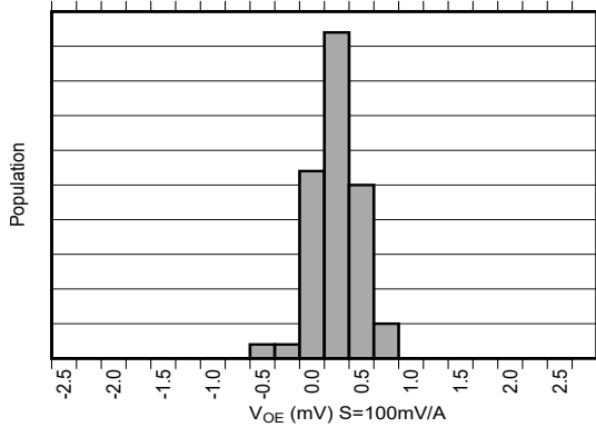
6-9. Offset Error Production Distribution
