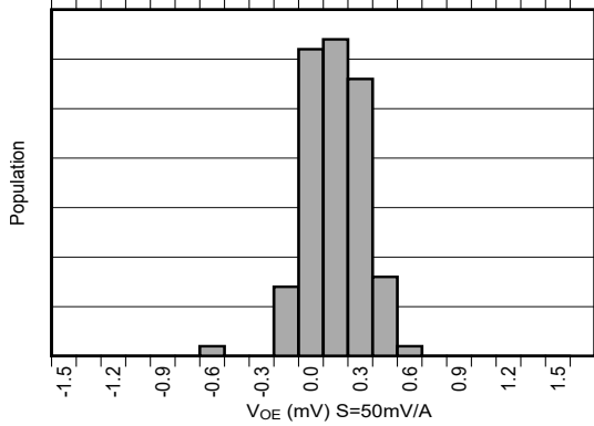
6-7. Offset Error Production Distribution
