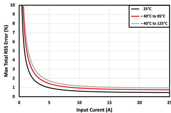
図 9-1. RSS Error vs Input Current
