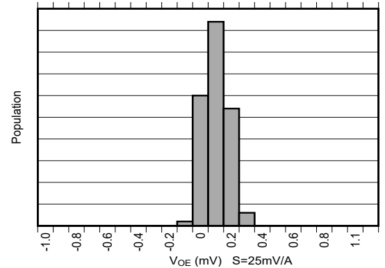
6-6. Offset Error Production Distribution
