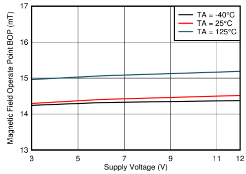
7-20. B OP vs V CC
