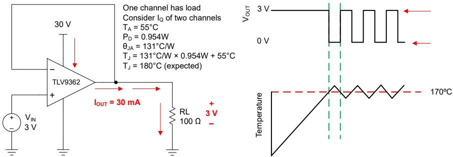
图 6-2. Thermal Protection
