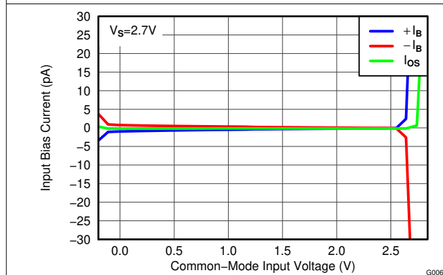
図 6-9. 入力バイアスおよび入力オフセット電流と同相入力電圧との関係
