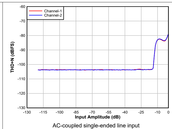
图 5-6. ADC THD+N Level vs Input
