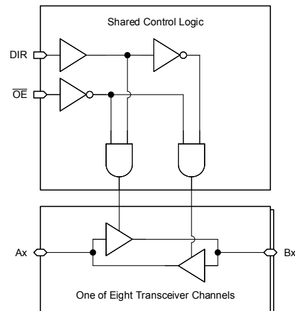
概略論理図 (正論理)
