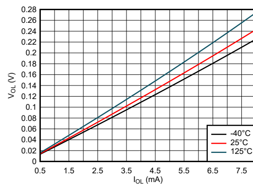
図 5-10. Low 状態における出力電圧と電流との関係、1.8V 電源
