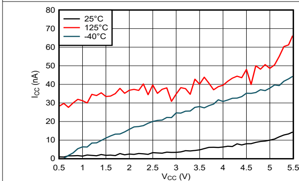
図 5-3. 電源電流と電源電圧との関係
