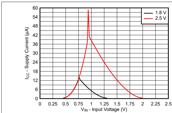
図 5-1. 入力電圧に対する電源電流、1.8V および 2.5V 電源
