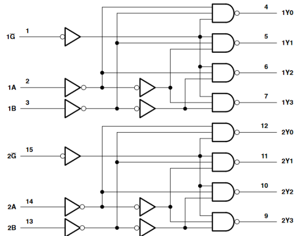
論理図 (正論理)
