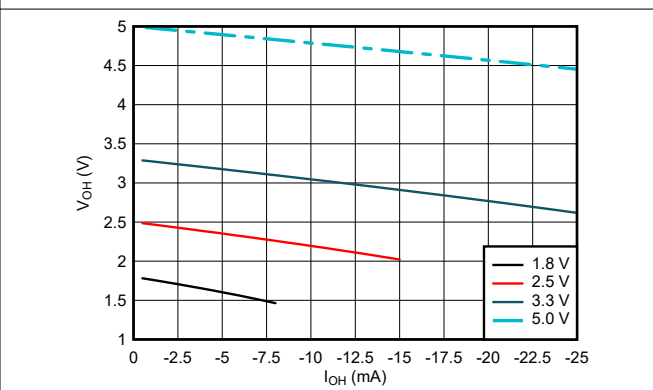
図 5-4. High 状態における出力電圧と電流との関係
