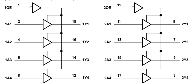
論理図 (正論理)
