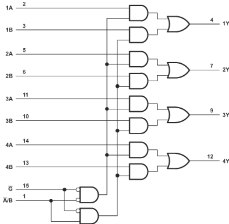
図 7-1. 論理図 (正論理)
