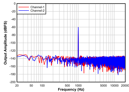
Plot12_MIC_FFT_m60dB.grf
