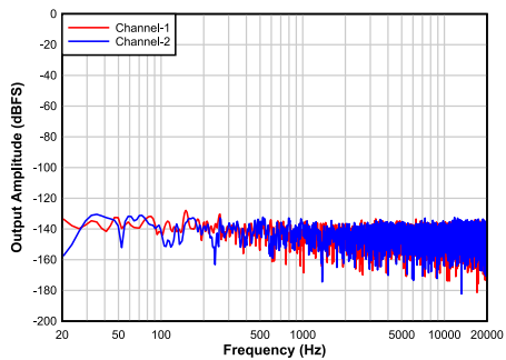
Plot11_MIC_FFT_IDLE.grf
